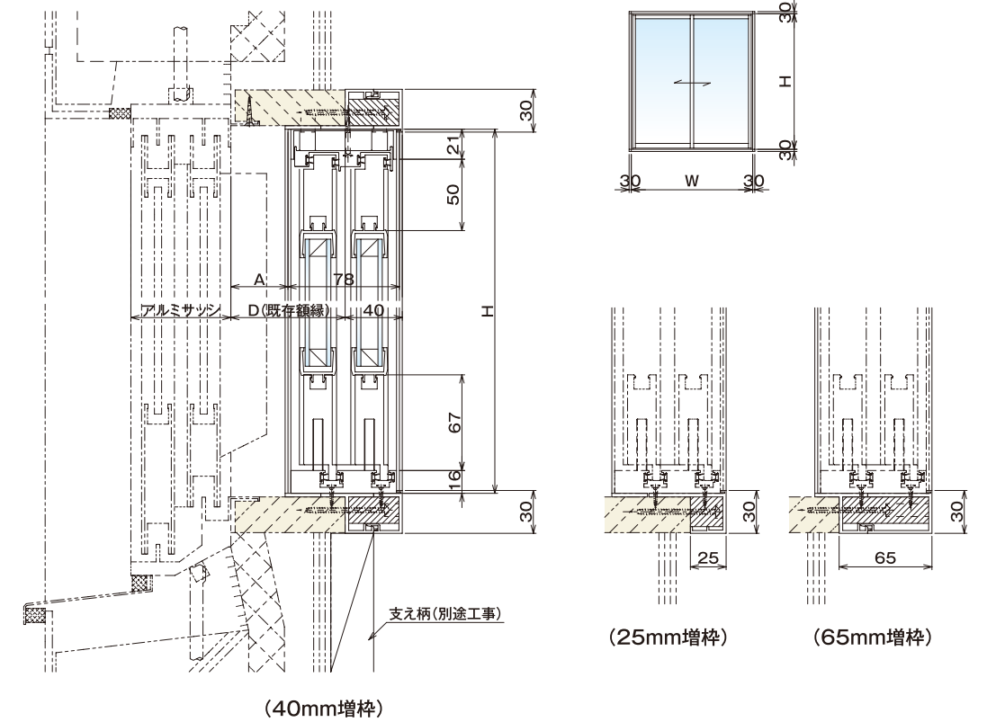
増枠 | 縦納まり図
