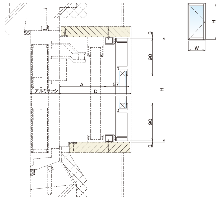
PDL型 | 縦納まり図
