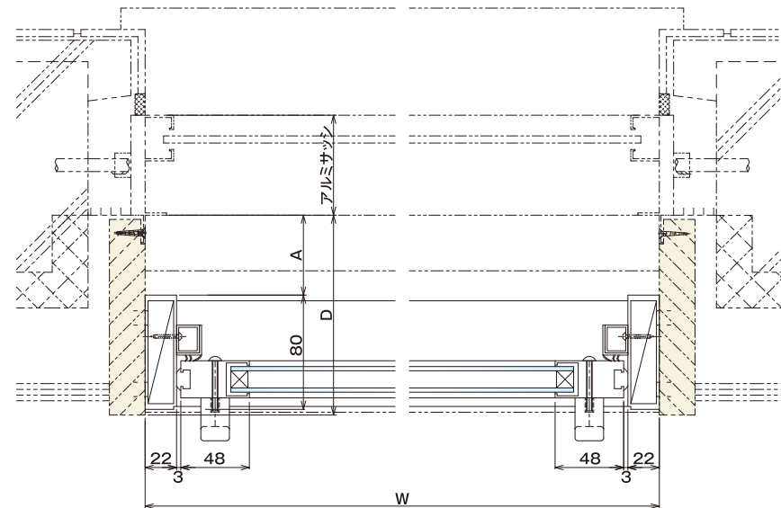
ケンドンNT型 | 横納まり図
