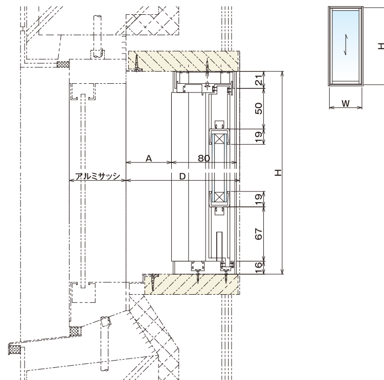
ケンドンNT型 | 縦納まり図
