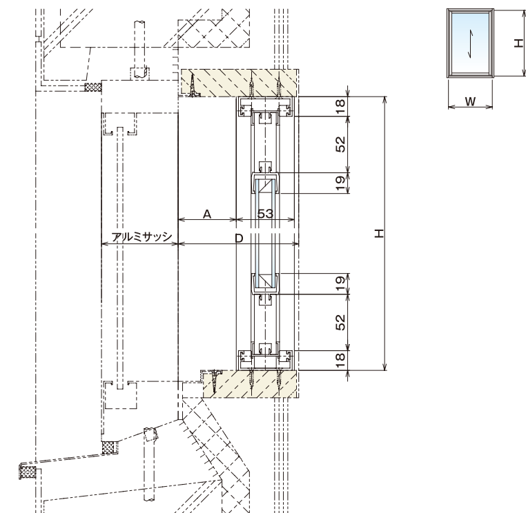
FKD型 | 縦納まり図
