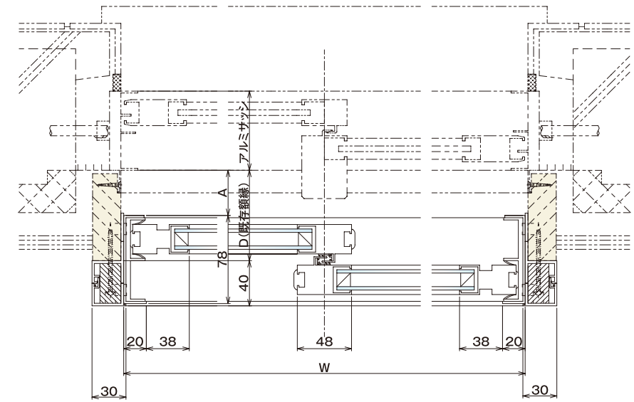
増枠(40mm) | 横納まり図
