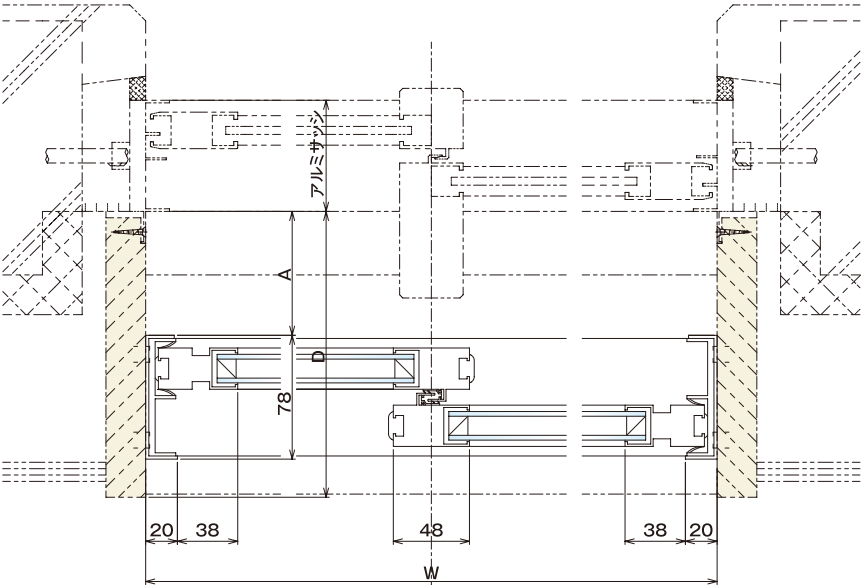
NT型・NTR型 | 横納まり図
