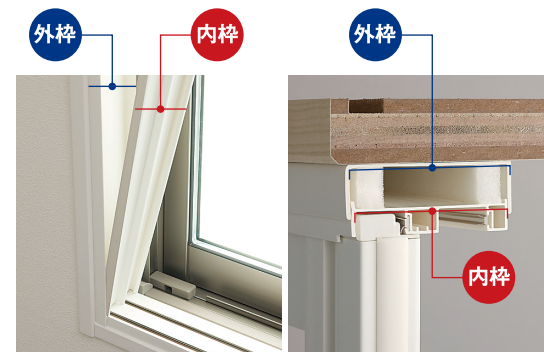
ダブルフレーム工法
