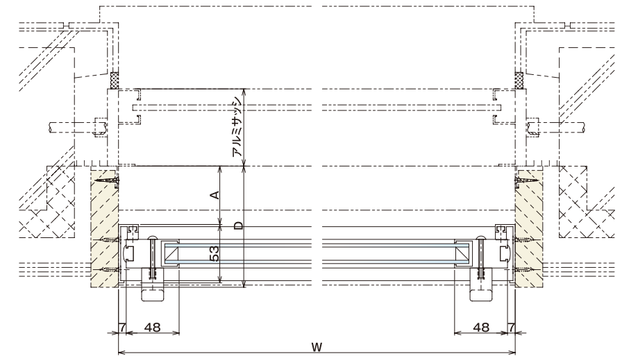
FKD型 | 横納まり図
