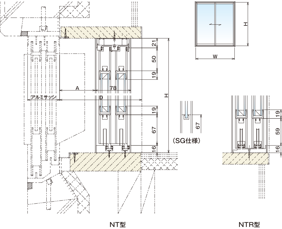
NT型・NTR型 | 縦納まり図
